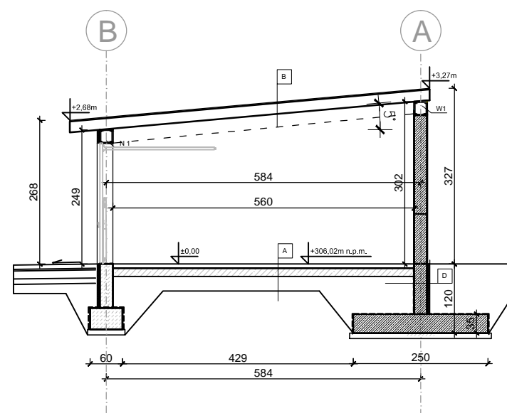
PRZEKRÓJ 2 SEGMENT
